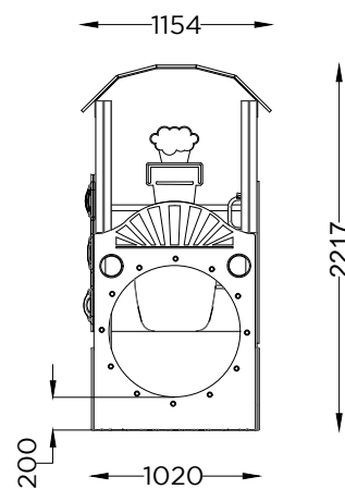
ALÇADO FRONTAL FRONT VIEW
