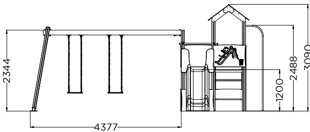
ALÇADO LATERAL SIDE VIEW
