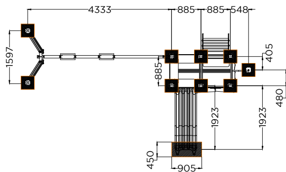
PLANTA . ESQUEMA DE FIXAÇÃO PLAN . INSTALLATION PLAN
