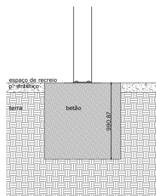
Fixação sobre Maciço de Betão
