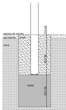
Fixação por Enterramento
