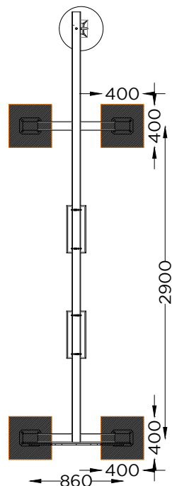
PLANTA . ESQUEMA DE FIXAÇÃO PLAN . INSTALLATION PLAN
