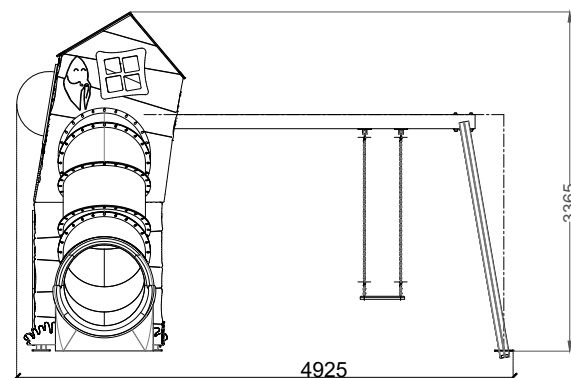
ALÇADO FRONTAL FRONT VIEW
