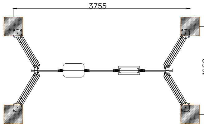
PLANTA . ESQUEMA DE FIXAÇÃO EM AREIA PLAN . SAND FIXATION SCHEME
