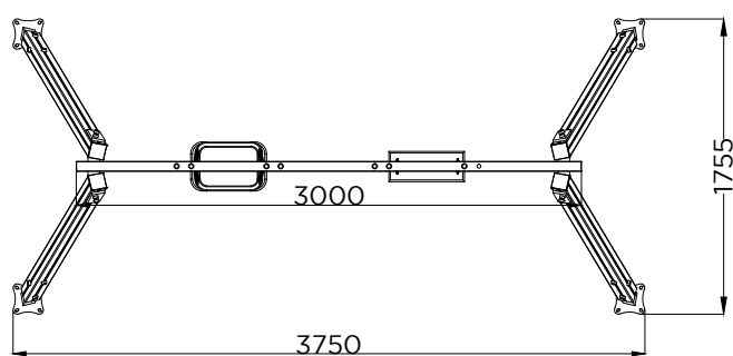
PLANTA PLAN
