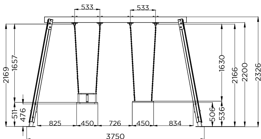
ALÇADO LATERAL SIDE VIEW
