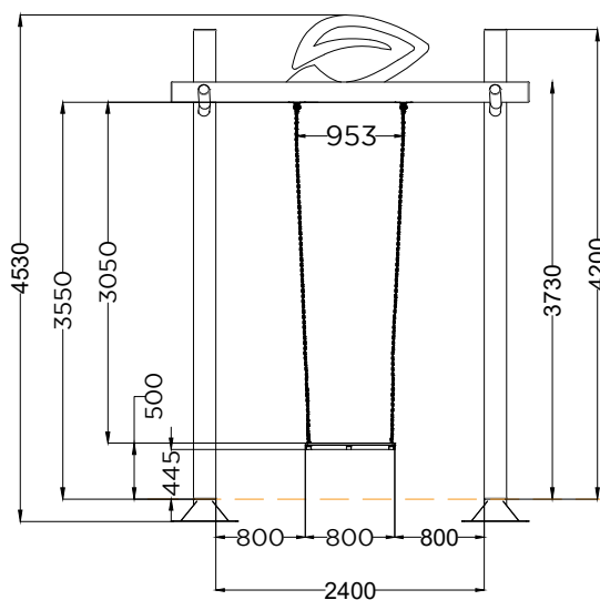
ALÇADO FRONTAL FRONT VIEW
