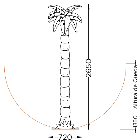
ALÇADO FRONTAL FRONT VIEW
