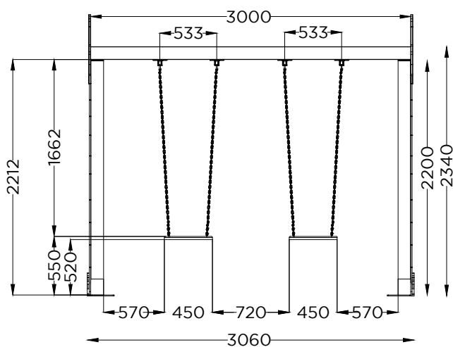
ALÇADO LATERAL SIDE VIEW
