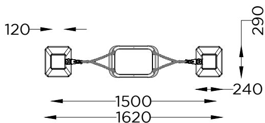
PLANTA PLAN
