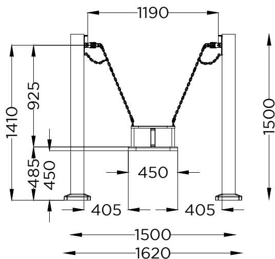
ALÇADO LATERAL SIDE VIEW
