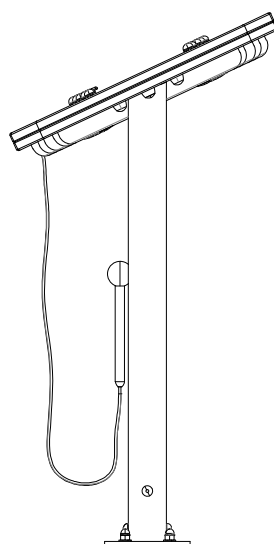
ALÇADO FRONTAL FRONT VIEW
