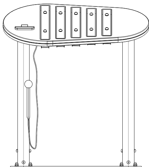
ALÇADO LATERAL SIDE VIEW
