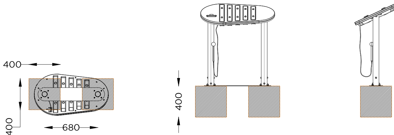
PLANTA . ESQUEMA DE FIXAÇÃO PLAN . INSTALLATION PLAN
