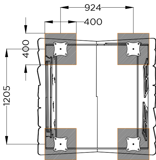
PLANTA . ESQUEMA DE FIXAÇÃO PLAN . INSTALLATION PLAN
