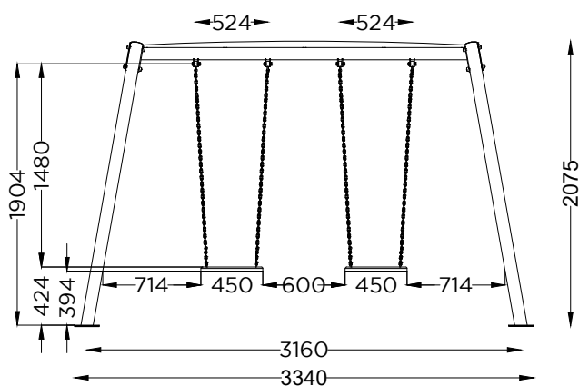
ALÇADO LATERAL SIDE VIEW
