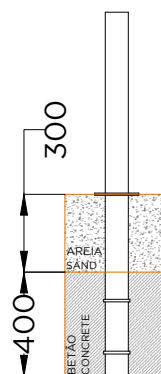
MACIÇO BETÃO + PISO AREIA P/ENTERRAMENTO CONCRETE BLOCK + SAND LAYER BY BURIAL
