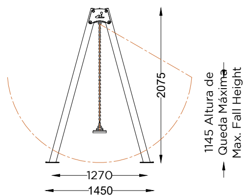
ALÇADO FRONTAL FRONT VIEW
