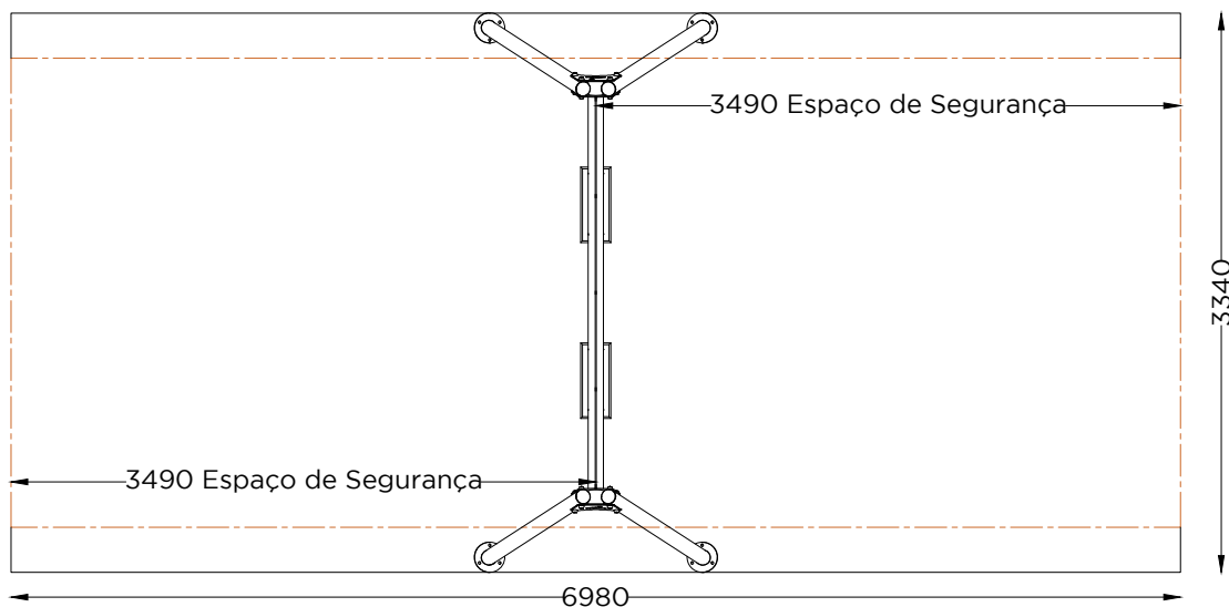
PLANTA - ESPAÇO DE SEGURANÇA NECESSÁRIO PLAN - SAFETY SPACE REQUIRED
