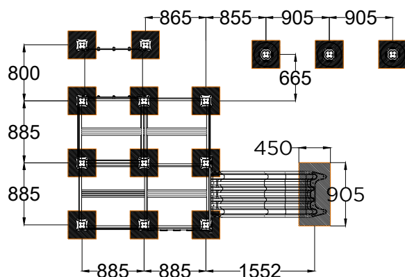
PLANTA . ESQUEMA DE FIXAÇÃO PLAN . INSTALLATION PLAN
