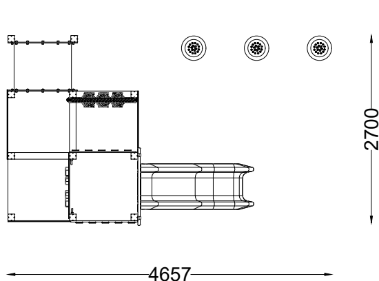
PLANTA PLAN
