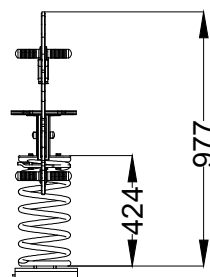
ALÇADO FRONTAL FRONT VIEW
