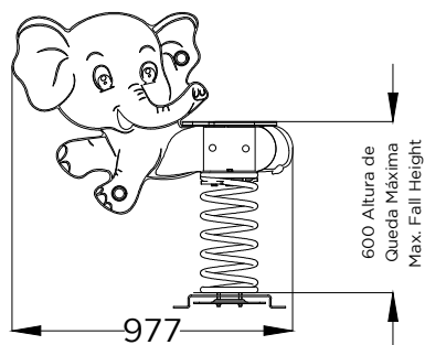
ALÇADO LATERAL SIDE VIEW
