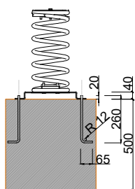
Alçado , Esquema de Fixação
