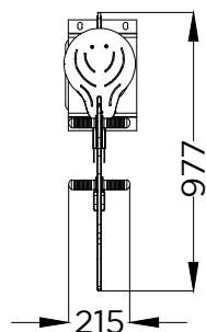
PLANTA PLAN
