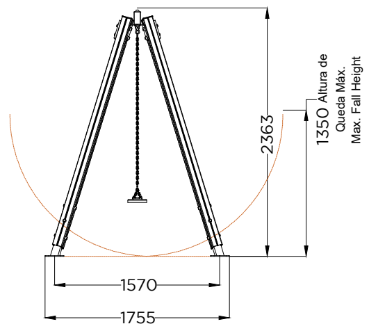
ALÇADO FRONTAL FRONT VIEW
