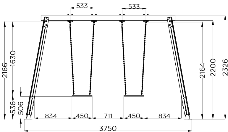
ALÇADO LATERAL SIDE VIEW
