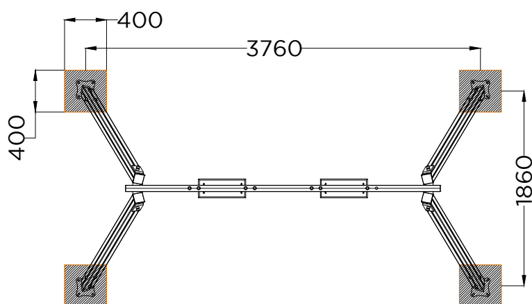
PLANTA . ESQUEMA DE FIXAÇÃO EM AREIA PLANT . SAND FIXATION SCHEME
