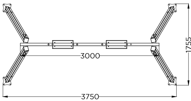
PLANTA PLAN
