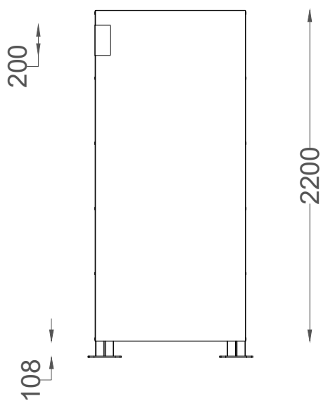
ALÇADO FRONTAL FRONT VIEW
