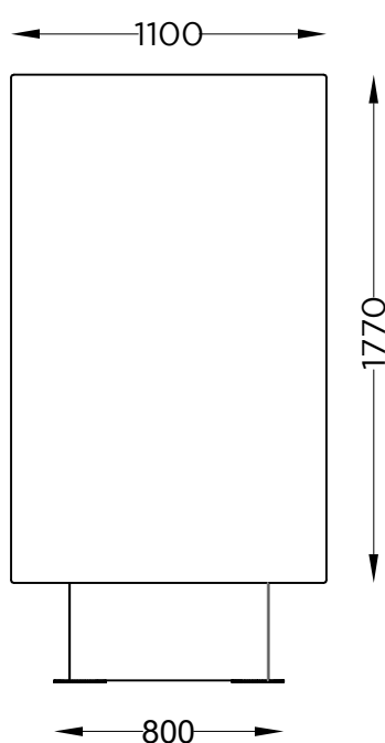
ALÇADO FRONTAL FRONT VIEW
