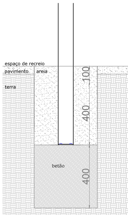
ESQUEMA DE FIXAÇÃO POR ENTERRAMENTO
