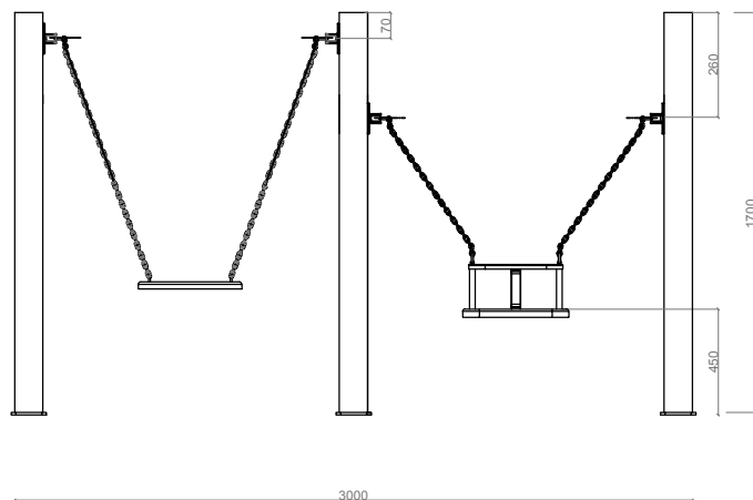
ALÇADO FRONTAL
