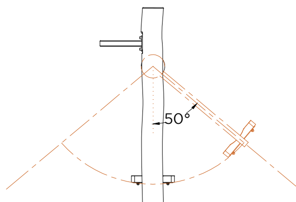
ALÇADO FRONTAL FRONT VIEW
