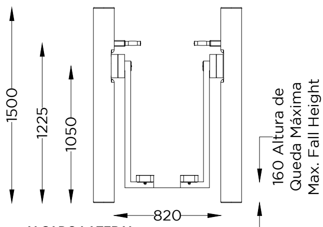
ALÇADO LATERAL SIDE VIEW
