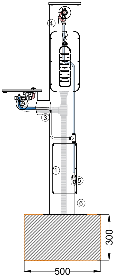
ALÇADO FRONTAL FRONT VIEW
