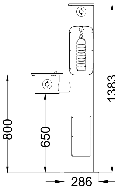
ALÇADO FRONTAL FRONT VIEW
