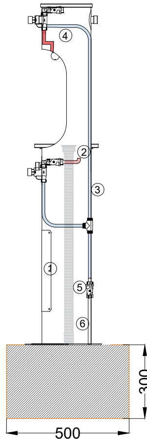
ALÇADO LATERAL SIDE VIEW
