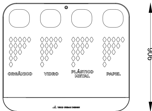
ALÇADO FRONTAL FRONT VIEW
