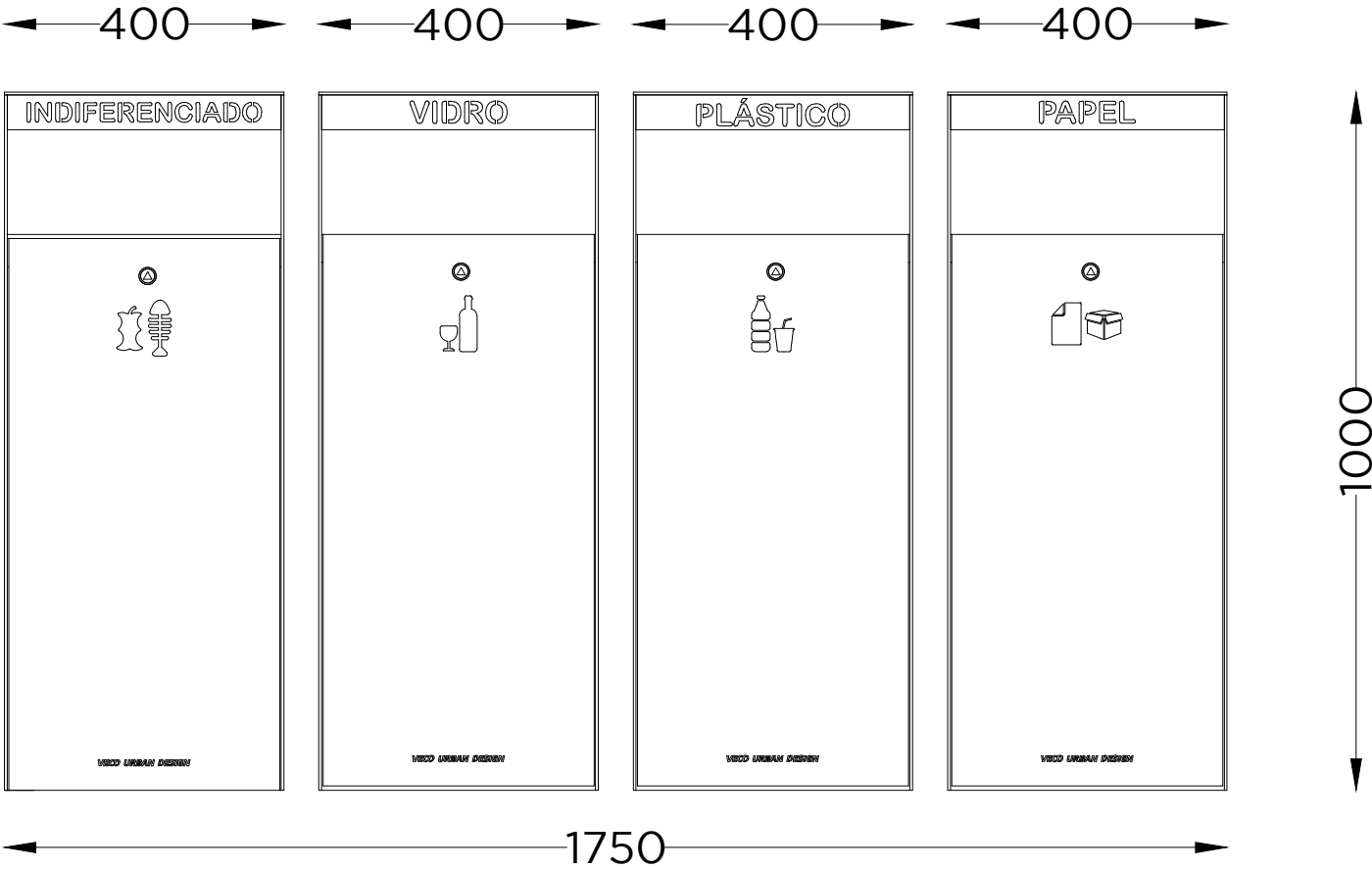
ALÇADO FRONTAL FRONT VIEW
