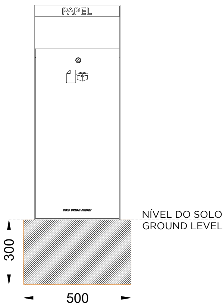
ALÇADO POSTERIOR . ESQUEMA DE FIXAÇÃO REAR VIEW . INSTALLATION PLAN
