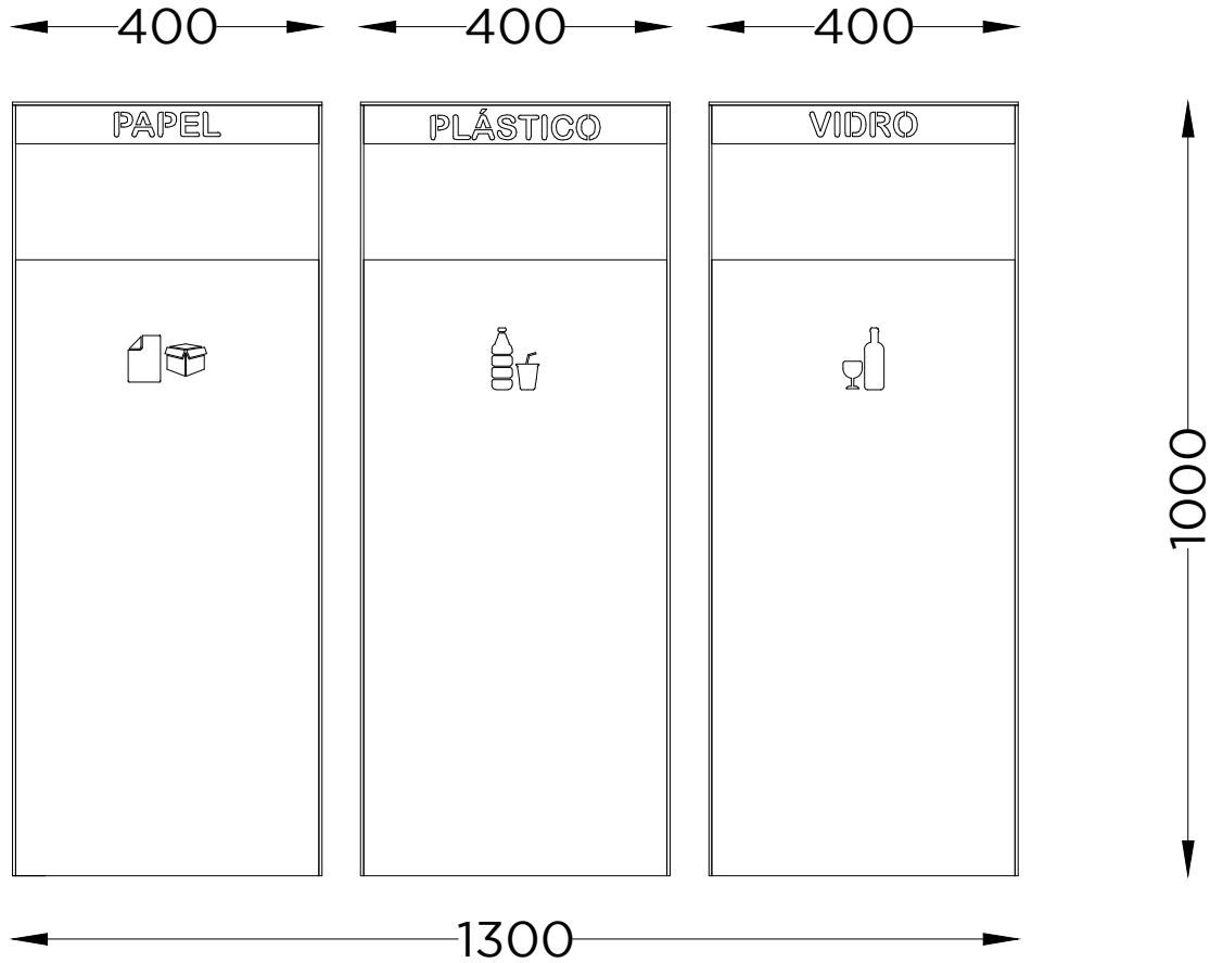
ALÇADO FRONTAL FRONT VIEW
