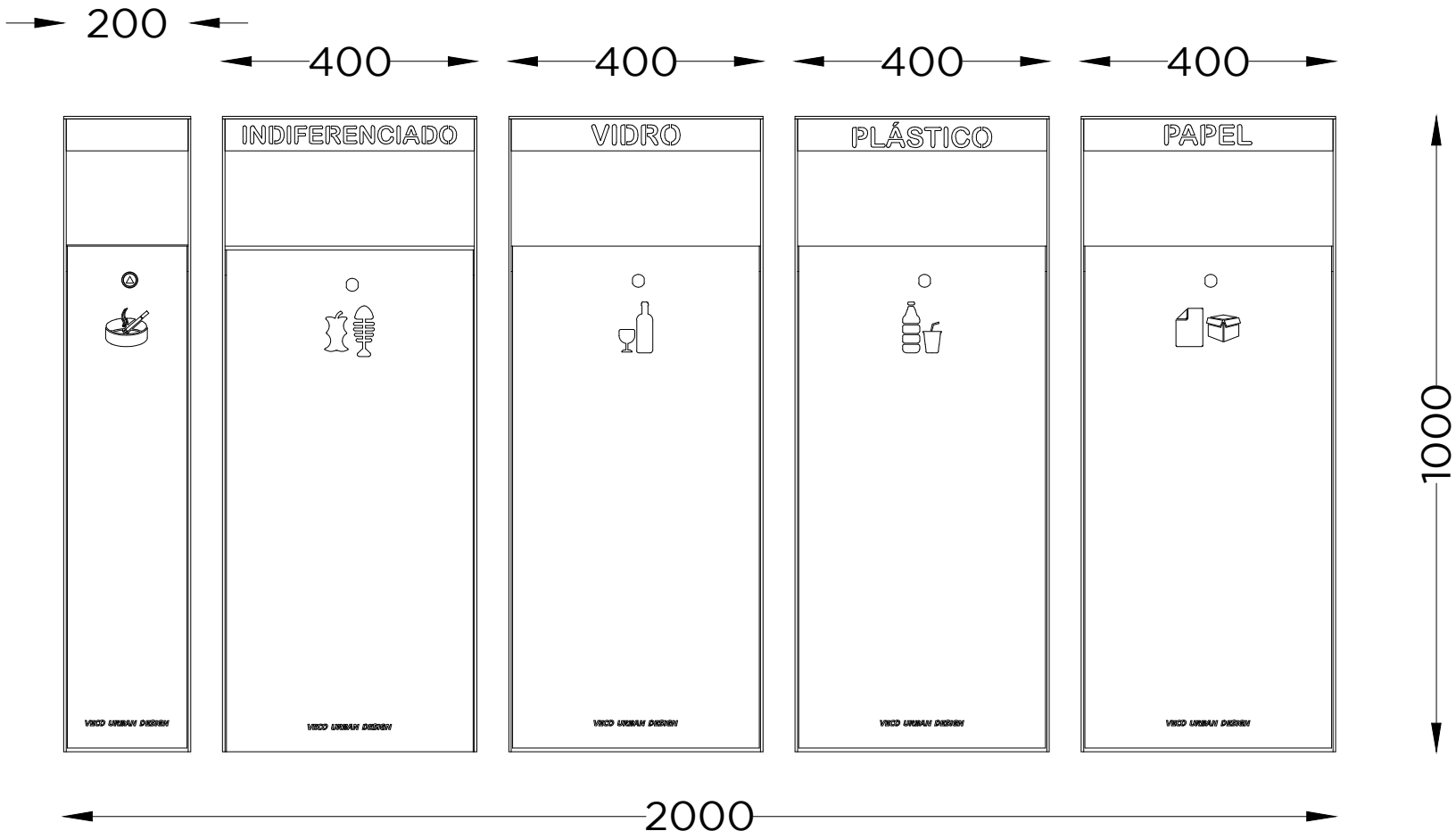
ALÇADO FRONTAL FRONT VIEW
