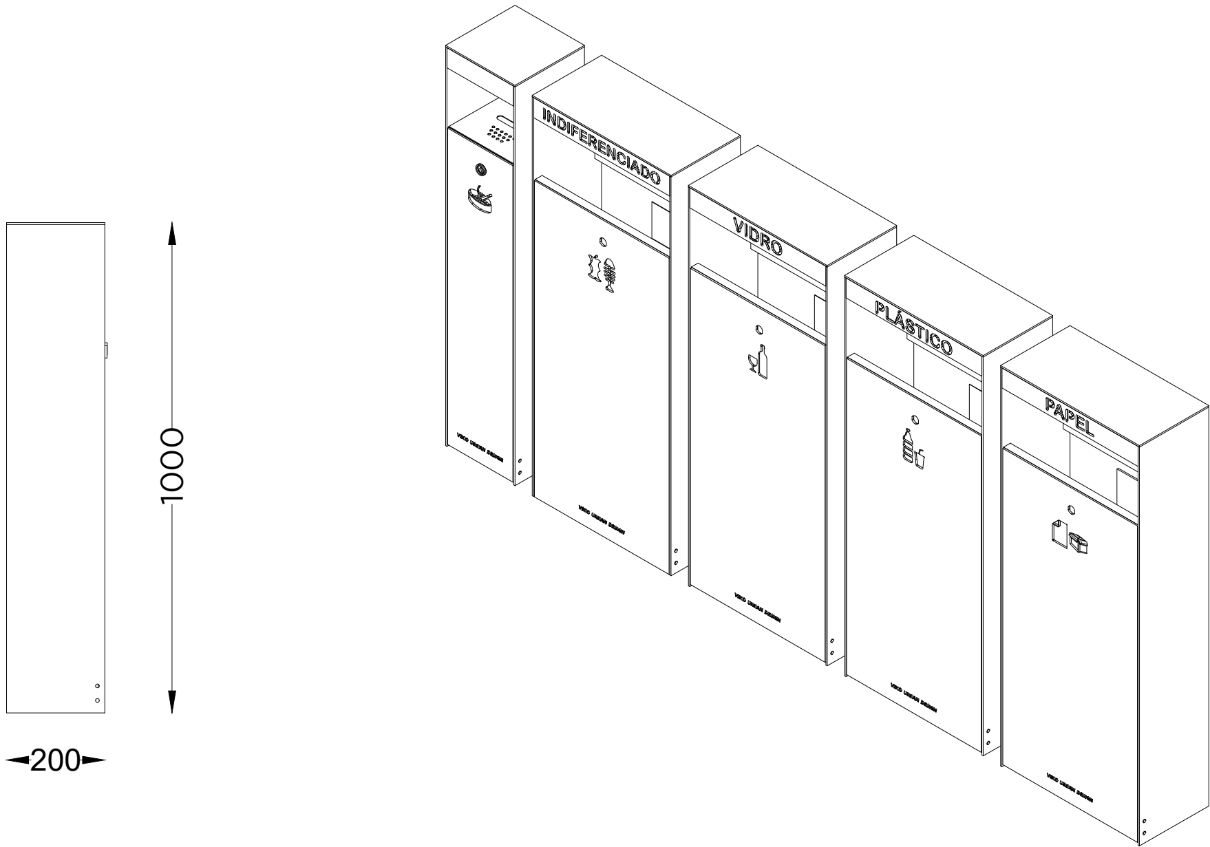
ALÇADO LATERAL SIDE VIEW
