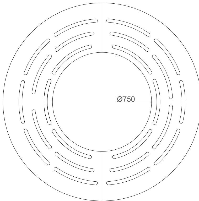
PLANTA PLAN
