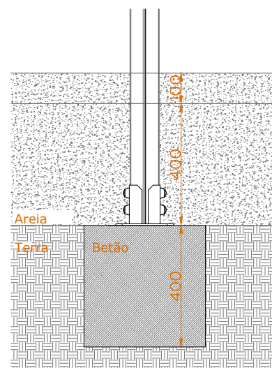
ESQUEMA DE FIXAÇÃO (PISO EM AREIA)
