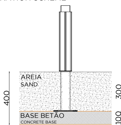
PLANTA . ESQUEMA DE FIXAÇÃO EM AREIA PLAN . SAND FIXATION SCHEME
