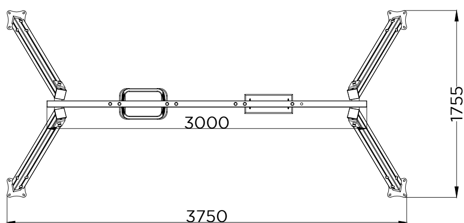
PLANTA PLAN
