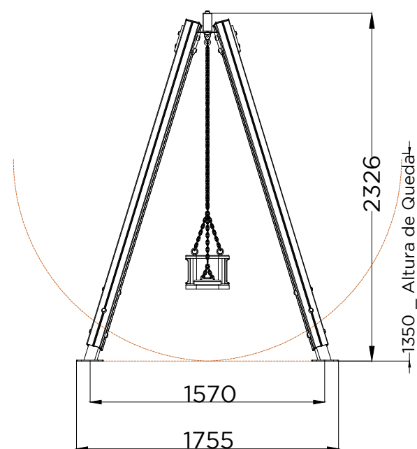
ALÇADO FRONTAL FRONT VIEW
