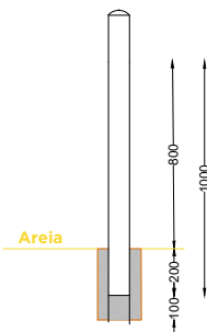
ESQUEMA DE FIXAÇÃO ENTERRAMENTO FIXATION SCHEME BURIAL
