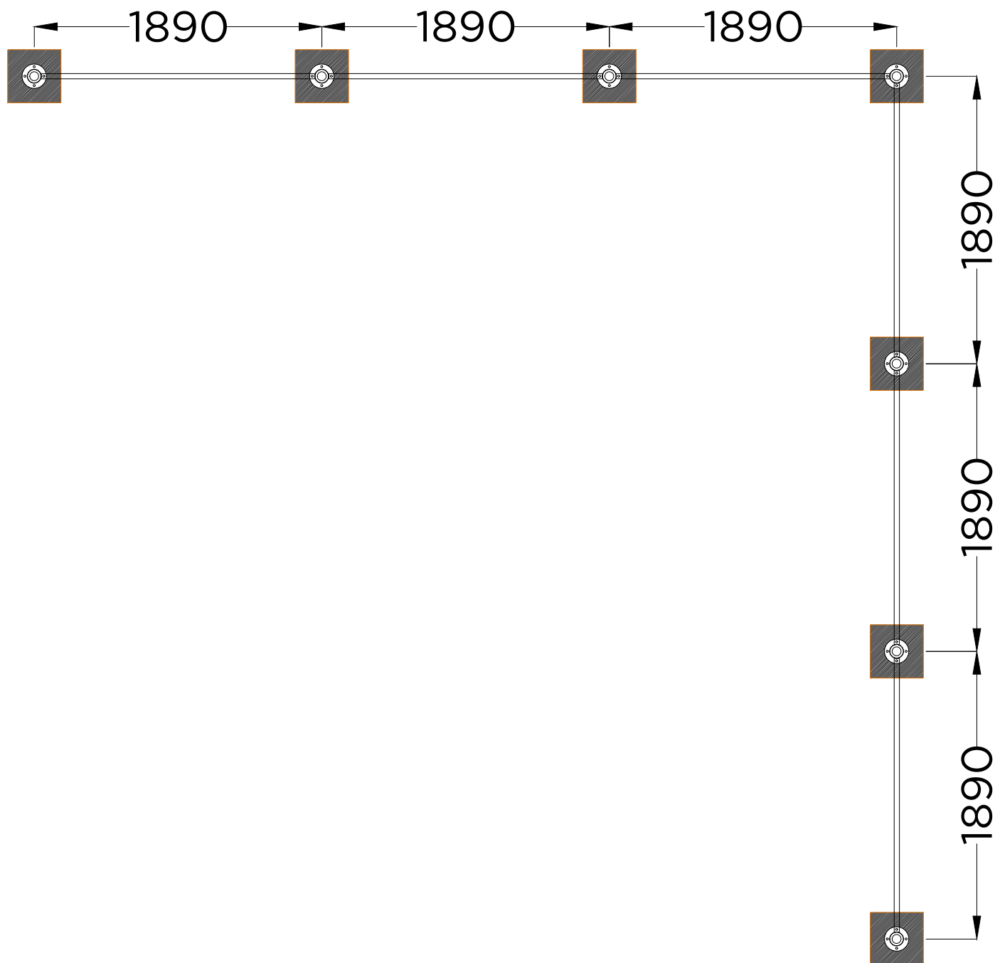
PLANTA . ESQUEMA DE FIXAÇÃO PLAN . INSTALLATION PLAN
