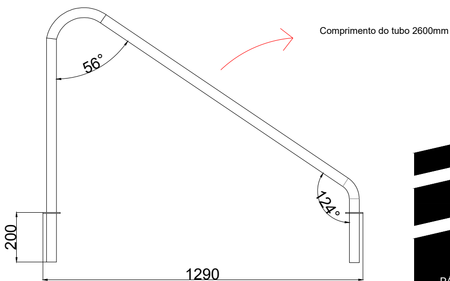
ALÇADO FRONTAL FRONT VIEW
