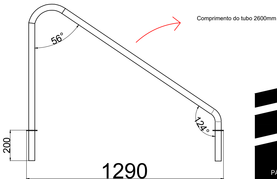
ALÇADO FRONTAL FRONT VIEW
