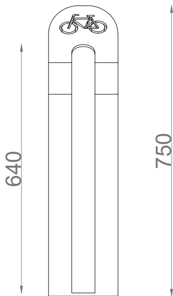
ALÇADO FRONTAL
