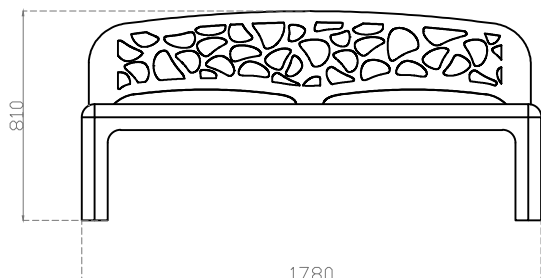
ALÇADO FRONTAL
