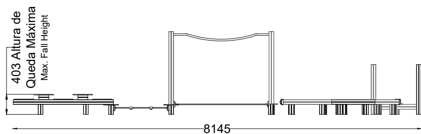
ALÇADO FRONTAL FRONT VIEW
