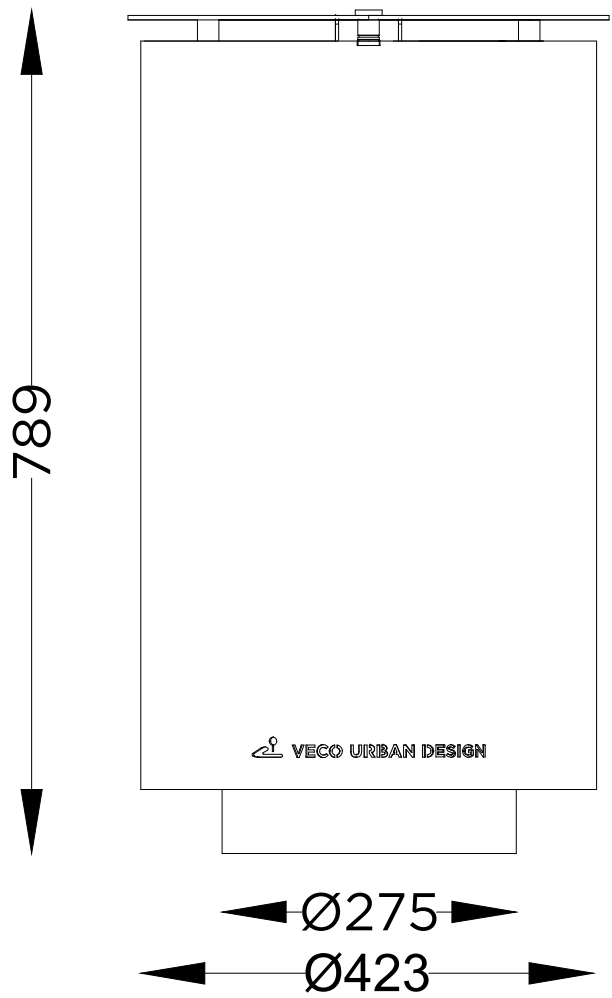
ALÇADO LATERAL SIDE VIEW
