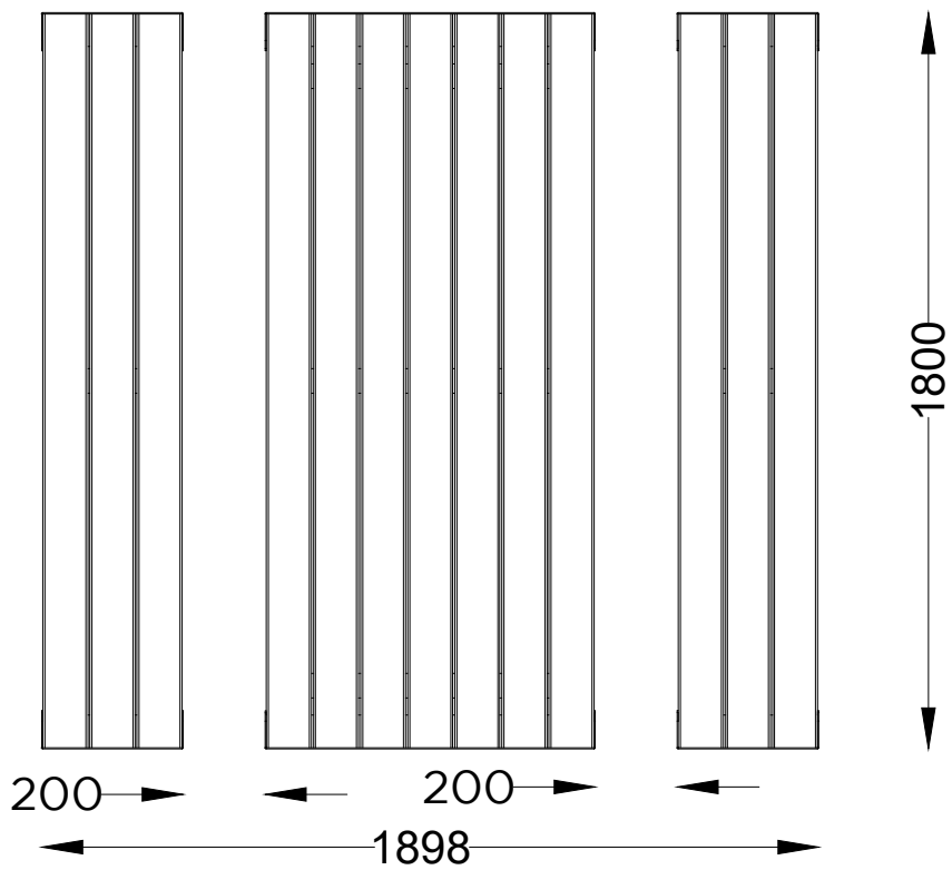
PLANTA PLAN
