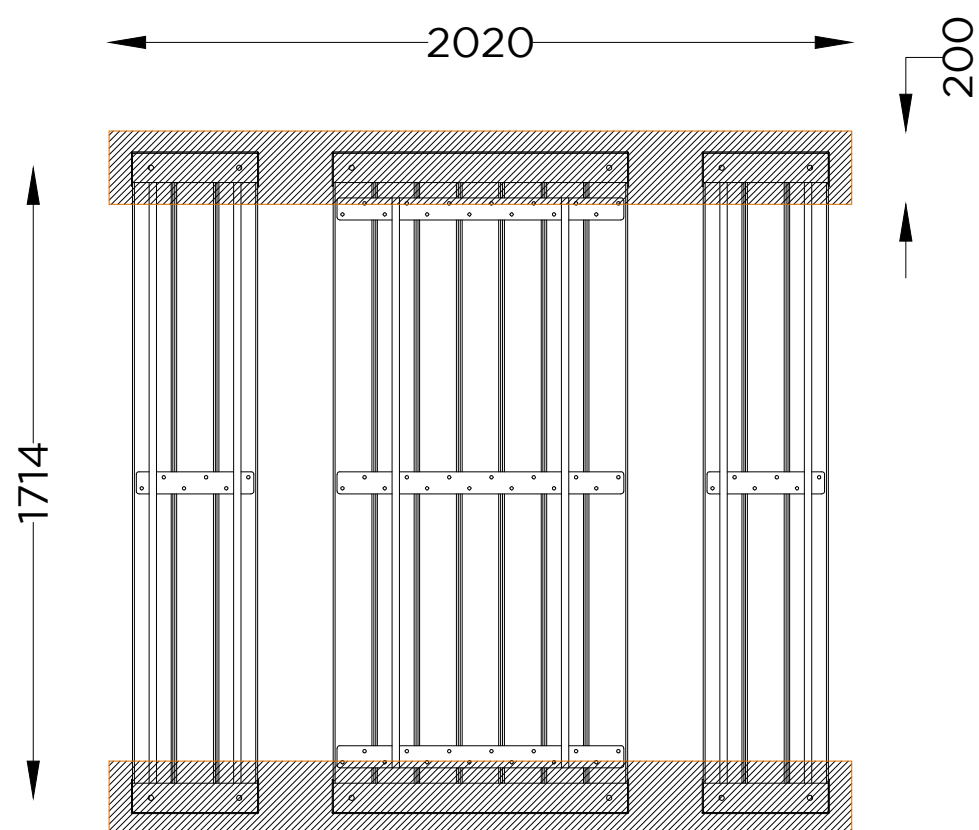
PLANTA . ESQUEMA DE FIXAÇÃO PLAN . INSTALLATION PLAN
