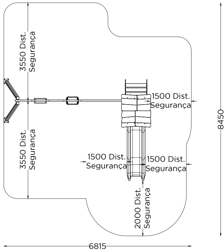
PLANTA - ESPAÇO DE SEGURANÇA NECESSÁRIO PLAN - SAFETY SPACE REQUIRED
