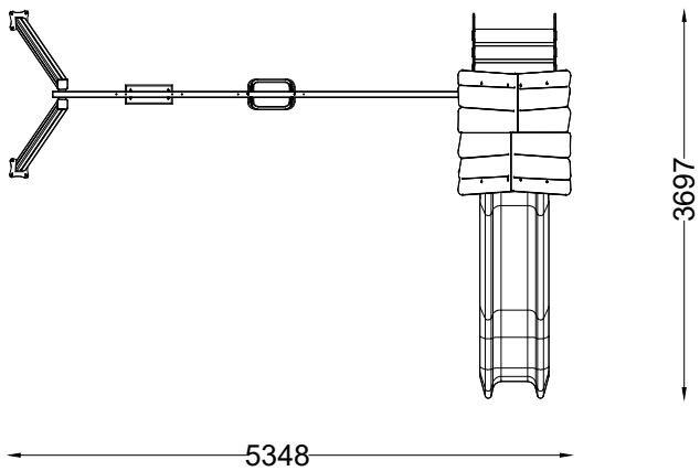
PLANTA PLAN
