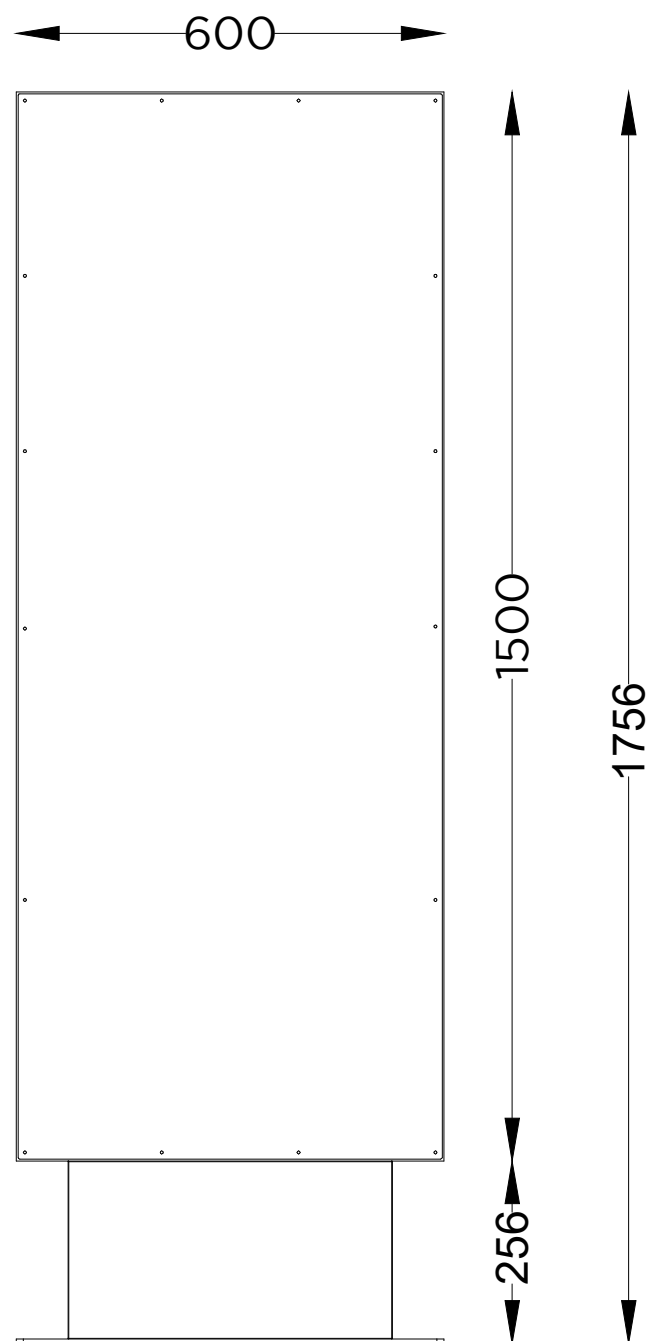
ALÇADO FRONTAL FRONT VIEW
