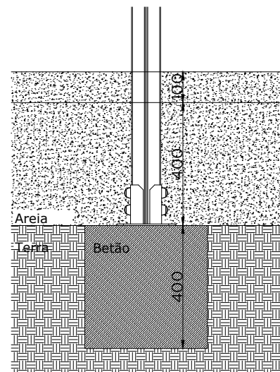
ESQUEMA DE FIXAÇÃO (PISO EM AREIA)
