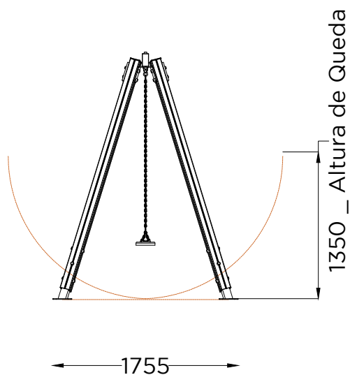
ALÇADO FRONTAL FRONT VIEW
