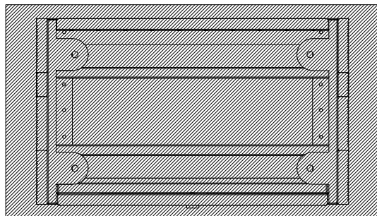
PLANTA . ESQUEMA DE FIXAÇÃO PLAN . INSTALLATION PLAN
