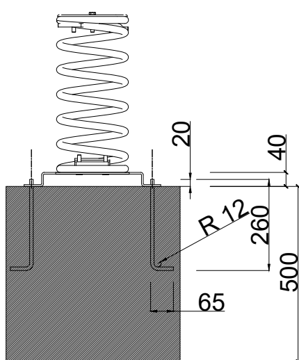
Alçado , Esquema de Fixação
