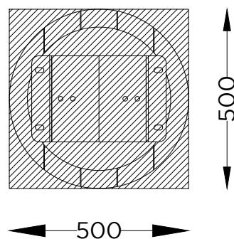
PLANTA, Esquema de Fixação
