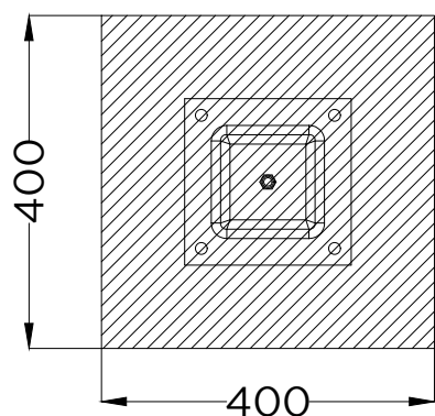
PLANTA . ESQUEMA DE FIXAÇÃO PLAN . INSTALLATION PLAN
