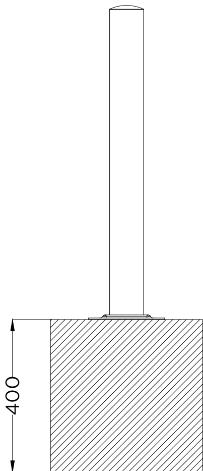
ALÇADO . ESQUEMA DO MACIÇO ALÇ. SCHEME OF THE MASSIVE
