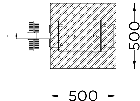
PLANTA, Esquema de Fixação
