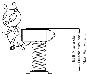
ALÇADO LATERAL SIDE VIEW
