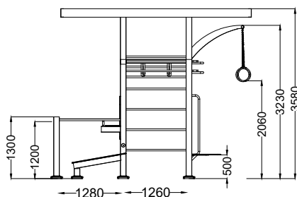
ALÇADO LATERAL SIDE VIEW
