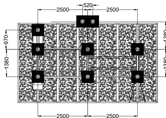
PLANTA . ESQUEMA DE FIXAÇÃO PLAN . INSTALLATION PLAN
