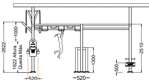
ALÇADO FRONTAL FRONT VIEW
