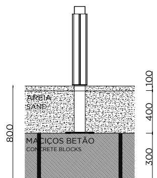
MACIÇOS BETÃO + PISO AREIA CONCRETE BLOCK + SAND LAYER
