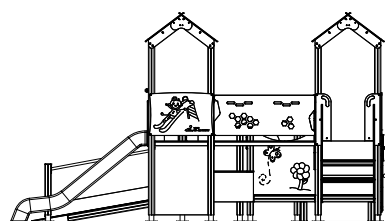
ALÇADO FRONTAL FRONT VIEW
