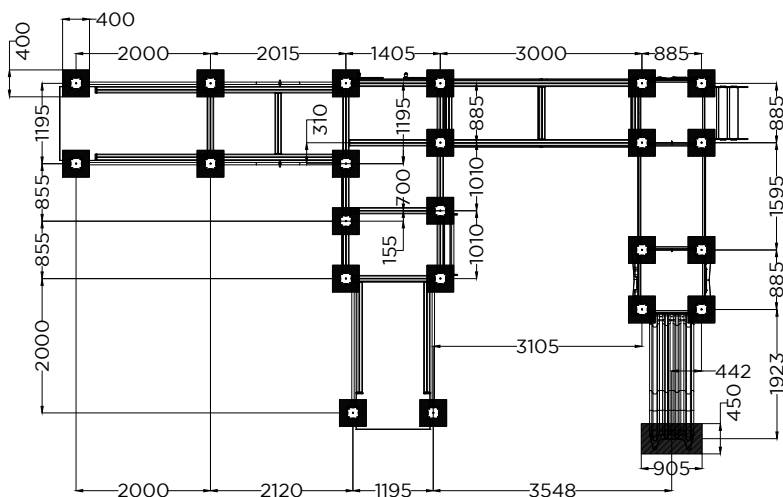
PLANTA . ESQUEMA DE FIXAÇÃO PLAN . INSTALLATION PLAN
