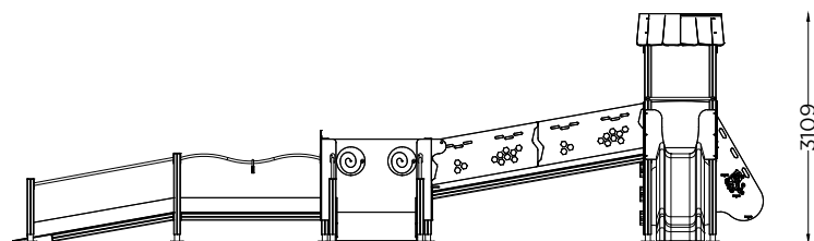
ALÇADO LATERAL SIDE VIEW
