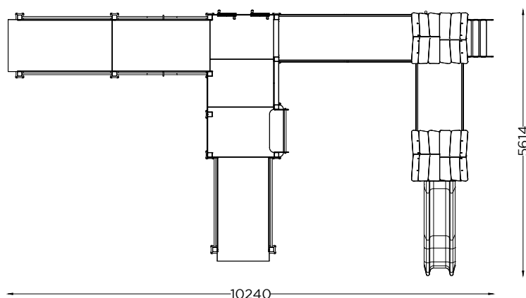
PLANTA PLAN
