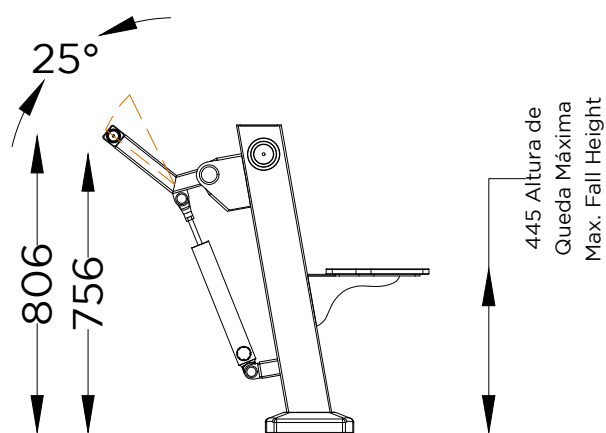
ALÇADO LATERAL SIDE VIEW
