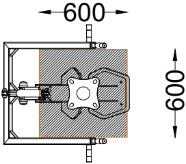
PLANTA . ESQUEMA DE FIXAÇÃO PLAN . INSTALLATION PLAN
