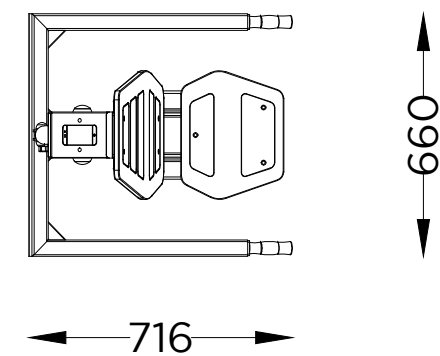
PLANTA PLAN
