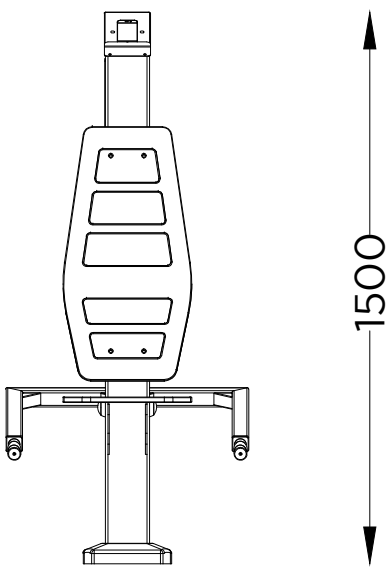
ALÇADO FRONTAL FRONT VIEW
