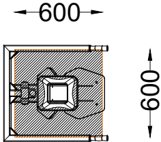
PLANTA . ESQUEMA DE FIXAÇÃO PLAN . INSTALLATION PLAN
