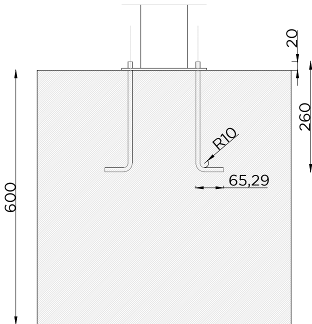
ALÇADO
