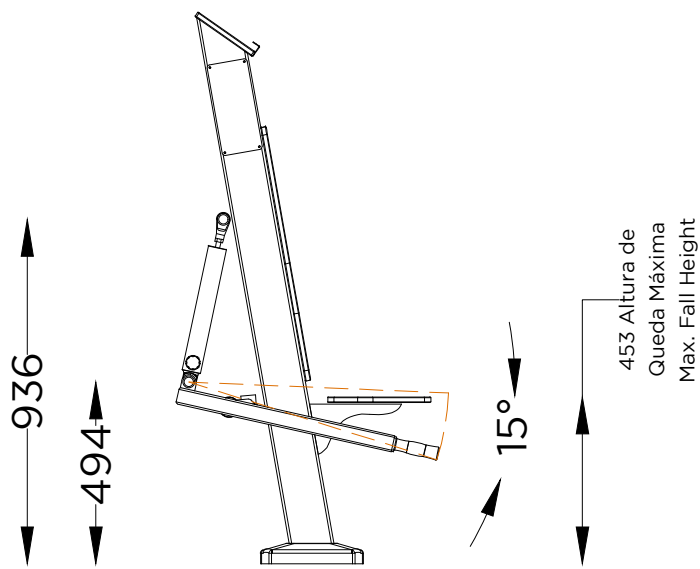
ALÇADO LATERAL SIDE VIEW
