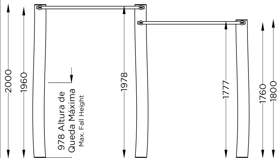
ALÇADO FRONTAL FRONT VIEW
