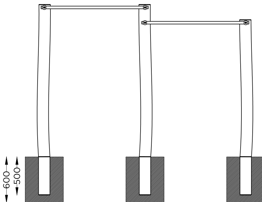
ALÇADO . ESQUEMA DE FIXAÇÃO SIDE VIEW . INSTALLATION PLAN
