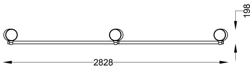
PLANTA - ESPAÇO DE SEGURANÇA NECESSÁRIO PLAN - SAFETY SPACE REQUIRED
