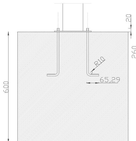
ALÇADO
