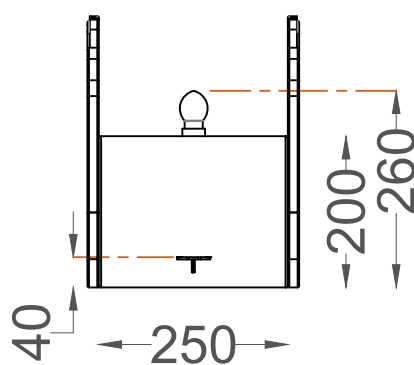
ALÇADO FRONTAL FRONT VIEW
